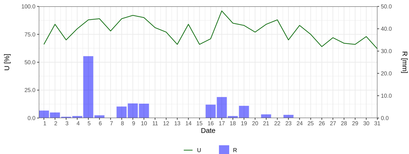
Ryc. 3. Średnia dobowa wilgotność względna powietrza i dobowe sumy opadu atmosferycznego Fig. 3. Mean daily relative humidity and daily sum of precipitation
