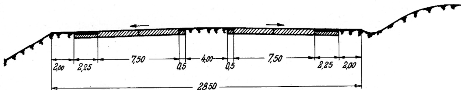
Bild 2. Der ab 1938 gültige Regelquerschnitt für Reichsautobahnen (RQ 28,5)
