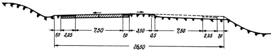
Bild 1. Besonderheit bei Reichsautobahnstrecken mit wenig Verkehr. RQ 26,5 mit nur einer ausgebauten Fahrbahn.
