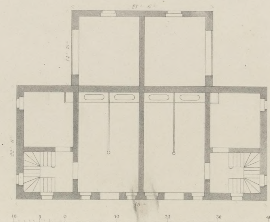
Stallgebäude in Klein-Glienecke bei Potsdam.
