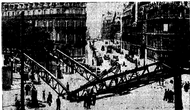
Wystawa paryska buduje się pod złym znakiem, bowiem nie tylko termin jej otwarcia odkłada się z dnia na dzień, ale oto most dla pieszych, wiodący na teren wystawowy — załamał się. Katastrofa, na szczęście wydrżyła się o takiej porze, że nikt z przechod- niów ani robotników nie odniósł szwanku.
