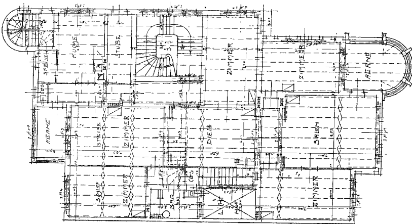
Grundriss vom Obergeschoss.
